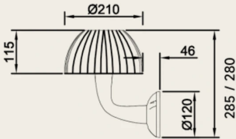
HV VERSION(E27)
