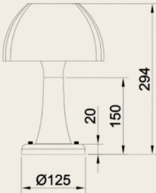
HV VERSION(E27)
