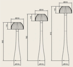
HV VERSION(E27)
