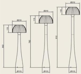
HV VERSION(E27)
